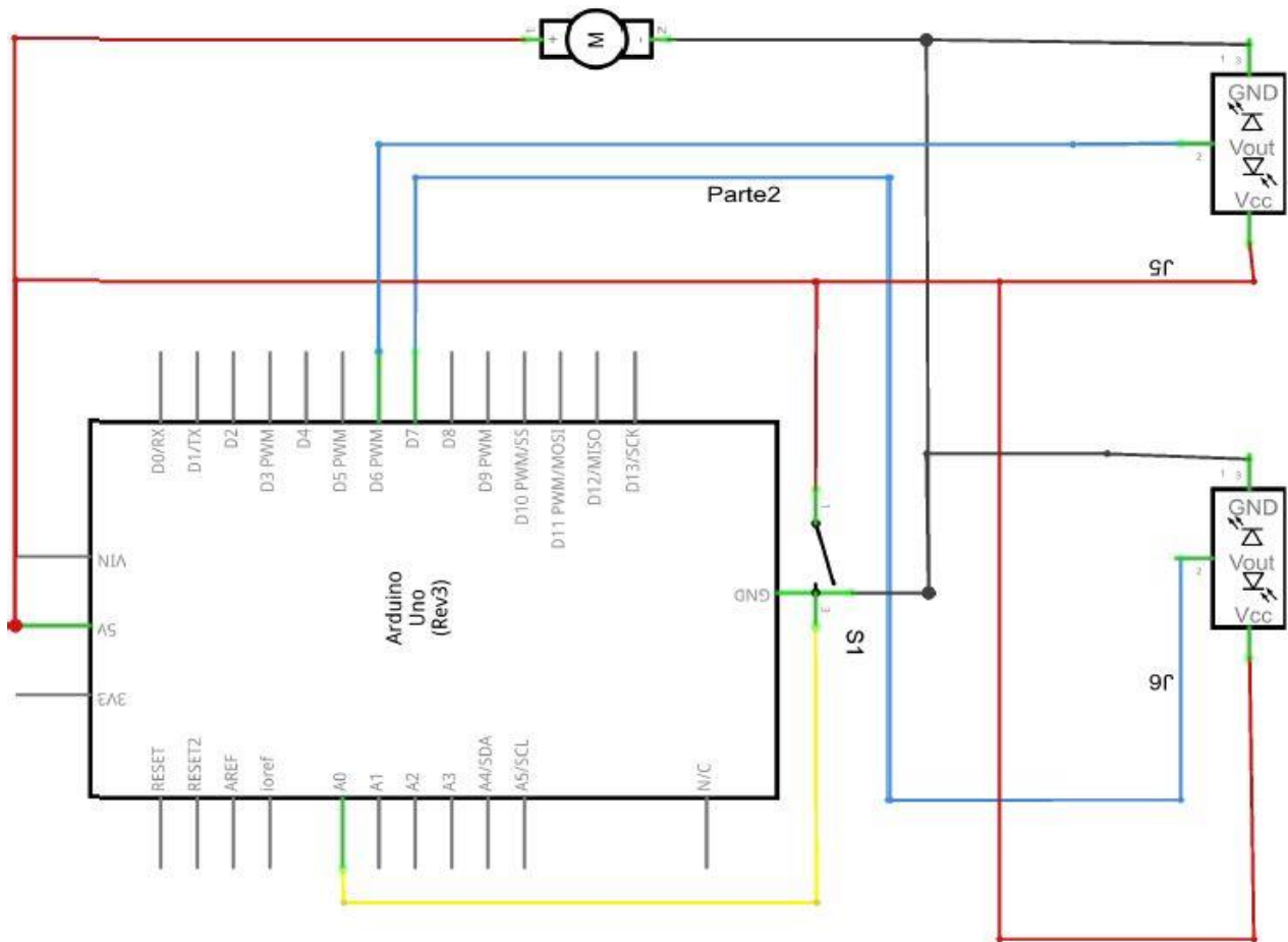
Fig. 51: Arduino Schematic
